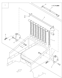
ETB-013174, Grabie łańcuchowe do nawozu
