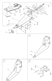
ETB-013119, Dyszel / wspornik do przesuwania
