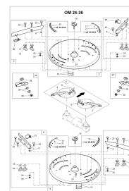
ETB-013153, Tarcza rozsiewająca OM 24-36
