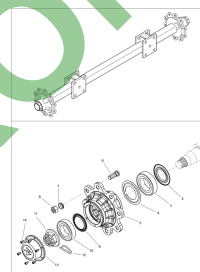
ETB-013124, Oś toczna
