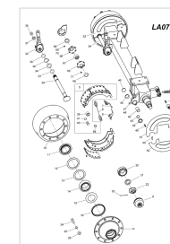
ETB-013125, Oś hamowana 25/40 km/h 10000 kg, rozstaw kół 1850 mm
