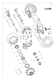
ETB-013126, Oś hamowana 25/40 km/h 10000 kg, rozstaw kół 2000 mm
