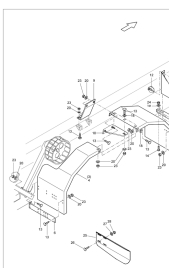
ETB-013164, Błotniki do ogumienia 700/50-26,5; 23.1-26 i 28L-26 bez napędu od koła jezdnego / z
