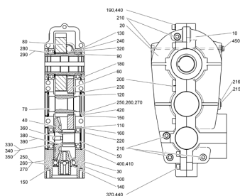
ETB-013138, Przekładnia ZG-B do pakietu wyposażenia "preciS" i "drive"
