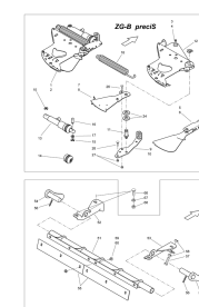
ETB-013141, Dna z otworami do skrzyni M / skrobak
