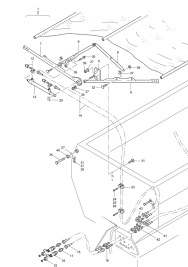
ETB-013173, Składana plandeka hydrauliczna
