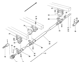
ETB-013118, Wałek napędu głównego
