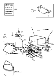
ETB-013151, Blacha kierująca
