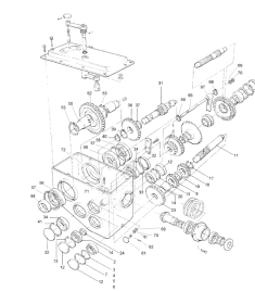
ETB-013137, Przekładnia, część 2
