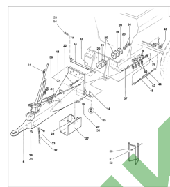
ETB-013120, Dyszel najazdowy
