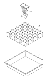
ETB-013176, Ruchome stanowisko pomiarowe
