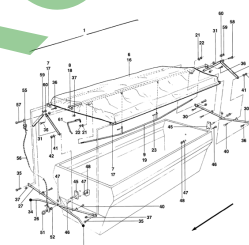
ETB-013172, Składana plandeka mechaniczna
