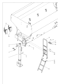
ETB-013122, Stopa podporowa; drabina; kliny pod koła
