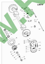
ETB-013127, Oś hamowana 25 km/h 8000 kg, rozstaw kół 1850 mm
