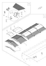
ETB-013123, Ruszty sitowe ZG-B 7001 ZG-B 10001
