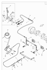
ETB-013131, Hydrauliczny układ hamulcowy solo, dwa siłowniki
