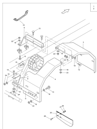
ETB-013166, Błotniki do ogumienia 550/60-22,5 i 600/55-26,5 / z napędem od koła jezdniego
