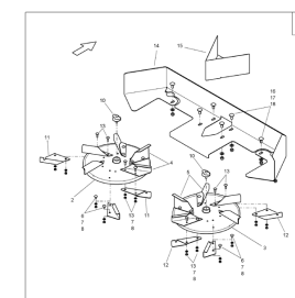
ETB-013154, Pakiet wyposażenia „Piasek”
