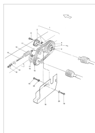
ETB-013134, Napęd pośredni do pakietu wyposażenia "Standard"
