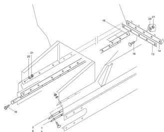
ETB-013142, Taśma uszczelniająca do skrzyni
