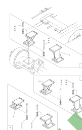
ETB-013132, Kocioł mocowania osi
