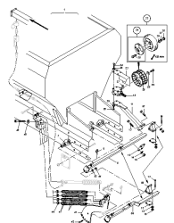
ETB-013170, Napęd od koła jezdniego, część 1
