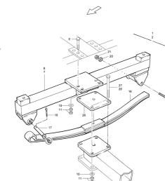
ETB-013133, zawieszenia
