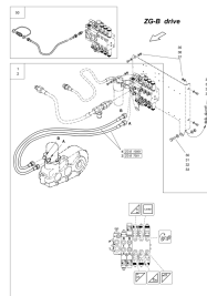
ETB-013156, Pakiet węży "napęd" / przewód sterujący wykrywający obciążenie
