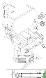
ETB-013171, Napęd od koła jezdniego, część 2
