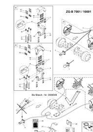
ETB-013161, Urządzenie do ważenia ZG-B
