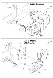
ETB-013135, Przekładnia do taśmy standardowej / preciS; drive
