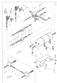
ETB-013130, Dwuobwodowy układ hamulcowy
