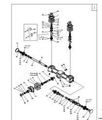
ETB-013149, Przekładnia rozdzielcza 540 obr./min, przełożenie 1:1,35 / 720 obr./min, przełożenie 1:1
