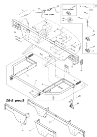
ETB-013147, Ściana tylna ramy / rurowy pałak ochronny / oświetlenie
