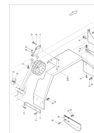
ETB-013165, Błotniki do ogumienia 23.1-26 i napędu od koła jezdnego
