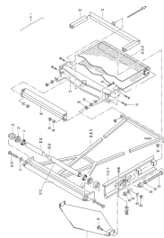
ETB-013143, Taśma, część 1
